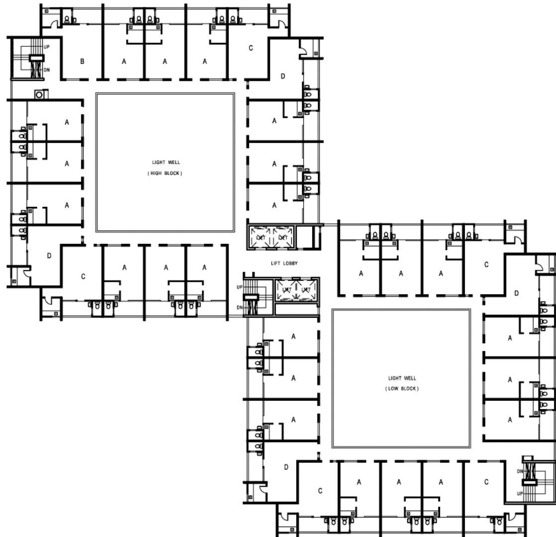
標準型大廈 雙塔式 標準樓層平面圖
